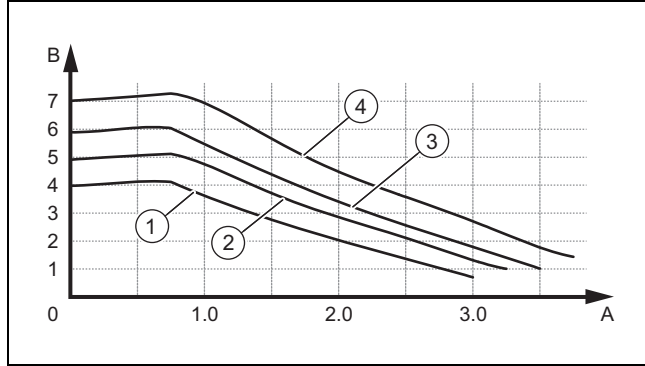
A Debi miktarı [Q (m³/san)] B Basma yüksekliği [m]
